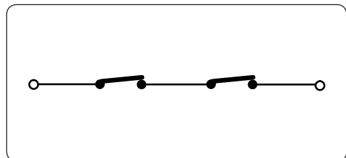
Fig. Conexión de 2 contactos N.C. en serie.
