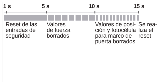
Fig. Sinopsis de la secuencia de tiempo del LED de estado (Status) en el carro al accionar el pulsador Reset verde
