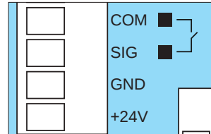
Borne de conexión para fotocélula de 4 hilos
