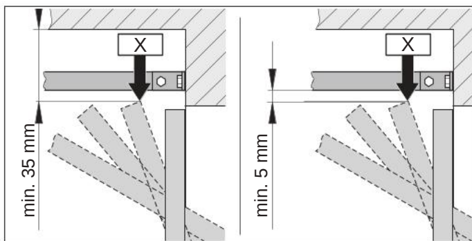
Fig. 1.1 para punto de altura máximo para puertas abatibles y puertas basculantes
